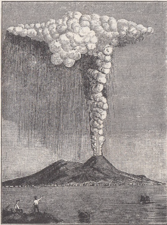
(رسم ۷۰) يانار طاغنىڭ فوتوروى.
