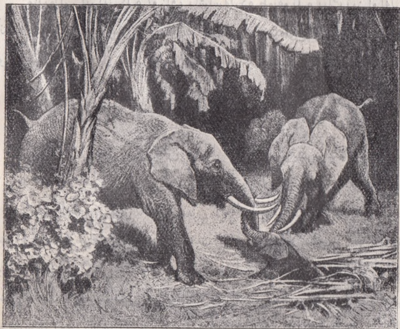
(رسم ۱۷). فیللر چوقورغه توشکان بالالارینی طارتوب چغارالر.
