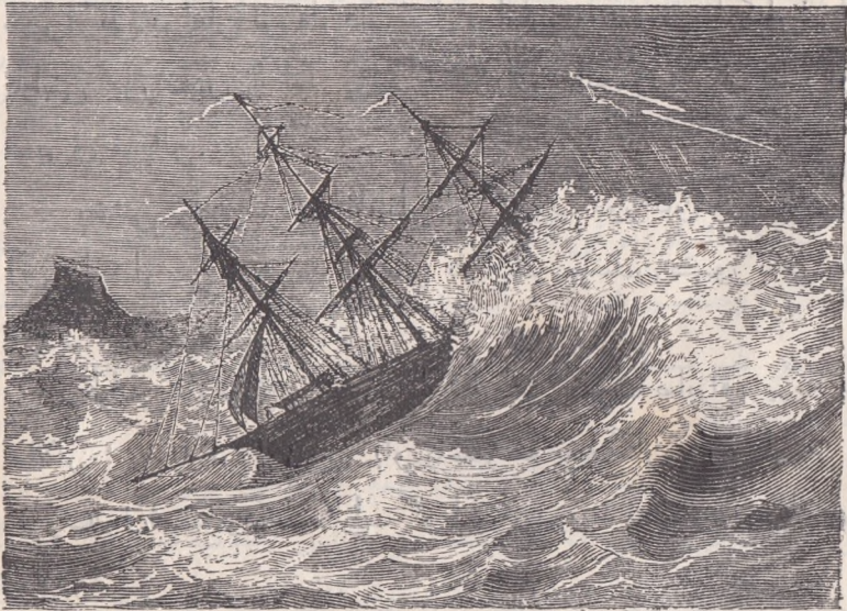
(رسم ۰۶۱) داؤلغه اوچوراغان کاراب.
