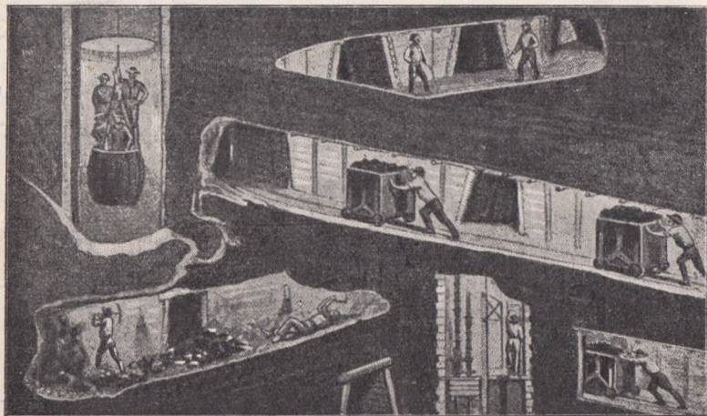
(رسم ۷۱. ) طاش کومر بازی.
