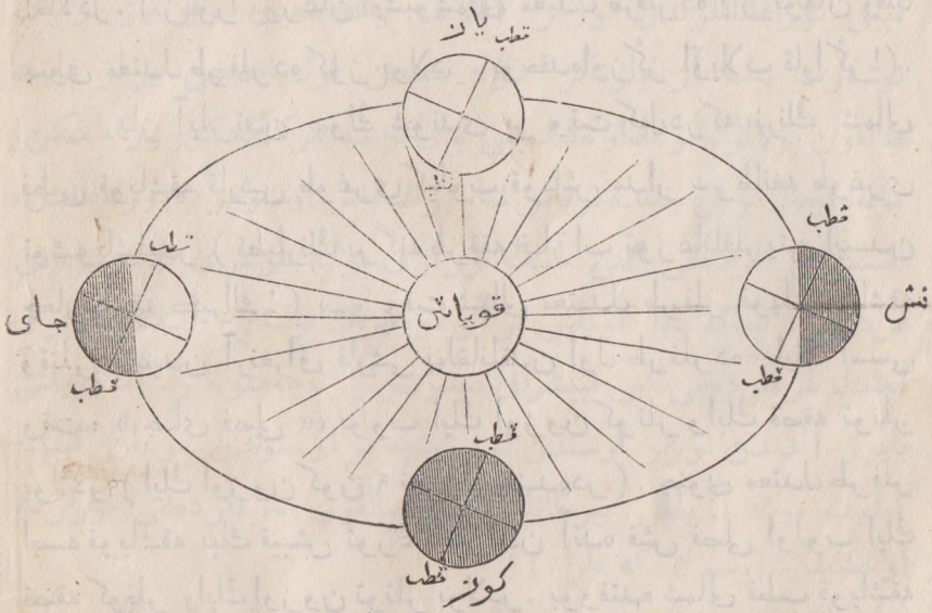
(رسم ۵). یرنڭ قویاش تیرەسندە آیله نوى ویلنڭ دورت وقتلری،
