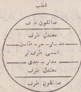
(رسم ۰۳) اسسی، معتدل و صالقون طرفلر هم قطبلر.
