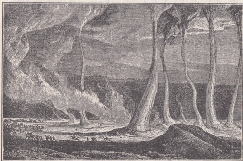
(رسم ۷۳ .) صحراى كىبرىدە قوم اۋىۋرمەسى .
