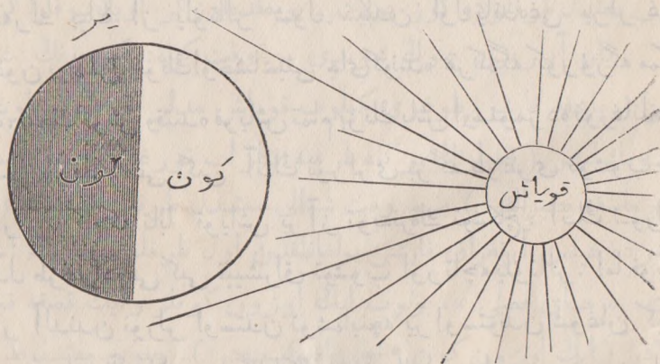
(رسم ۰۴) کون ایله تون نڭ حاصل بولوی .
