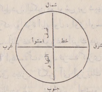
(رسم ۰۲) جهات اربعه، خط استوا و نصف النهار.
